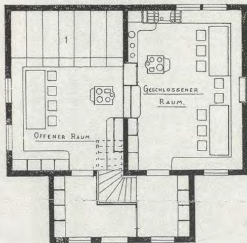
Erdgeschoss (offen und geschlossen).
