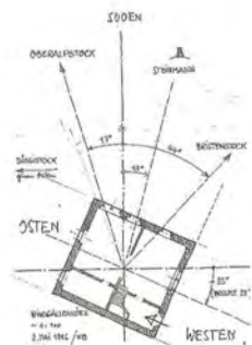
Heissdiskutierte Planunterlage für die Windgällenhütte
